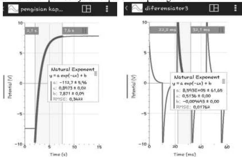
Gambar 4. Tampilankarakteristikkapasitor
