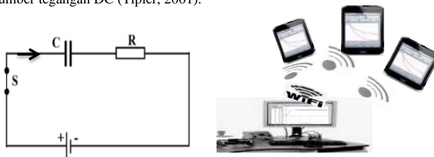
Gambar 2. Rangkaian percobaan
