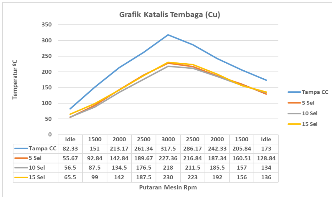
Gambar 7. Pengaruh putaran mesin terhadap temperatur pada Katalis Tembaga (Cu)
