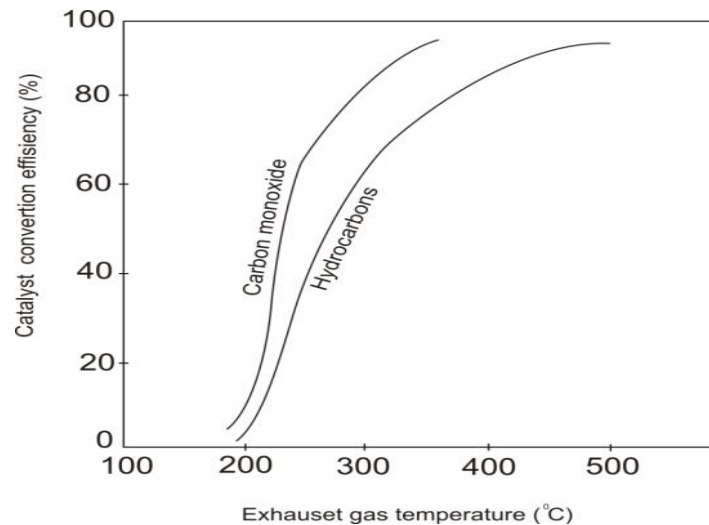
Gambar 2. Efisiensi Konversi CO Dan HC Berhubungan Dengan Temperature Gas Buang, [9]
