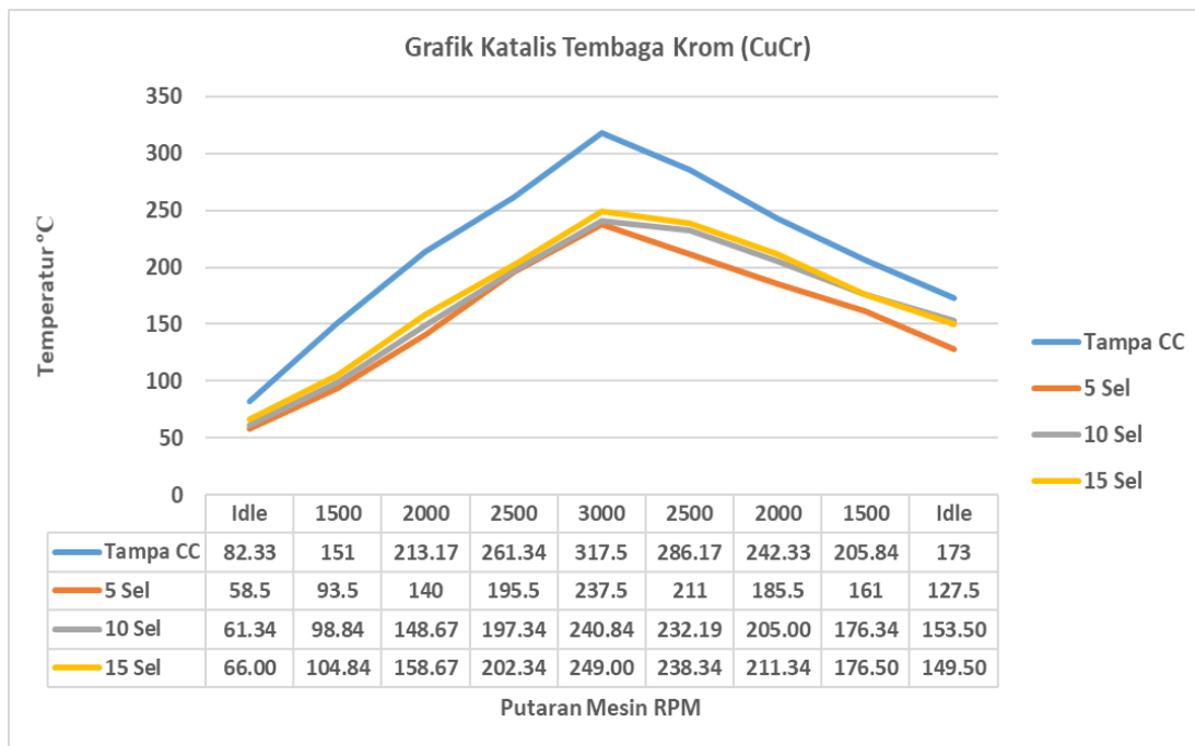
Gambar 8. Pengaruh putaran mesin terhadap temperatur pada Katalis Tembaga Krom (CuCr)
