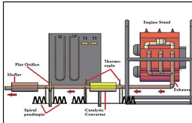
Gambar 6. Pengukuran Temperatur Pada Mesin Uji
